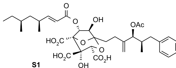
Fig. 2. Squalenstatin S1 .
